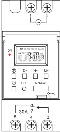
◆919s(30A)
