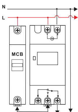
TM-919s(5P)30A
